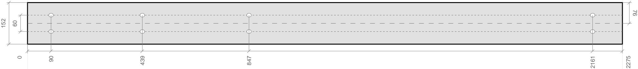
View B: 152 mm Web · Elevation · 60 mm Web Punch Spacing · 76 mm Center Line
